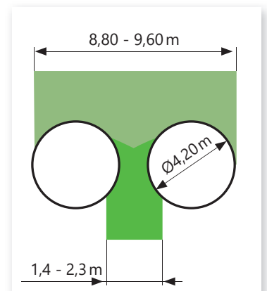
SP-962H zweirotoriger Schwader für Mittelschwade mit hydraulisch einstellbarer Arbeitsfläche Ergänzung des Hydraulikkreises durch Schösser im Standard
